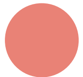
Alignement des investissements sur la taxinomie, hors obligations souveraines*
